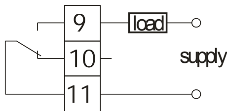
Fig. 6. Control/Alarm output
